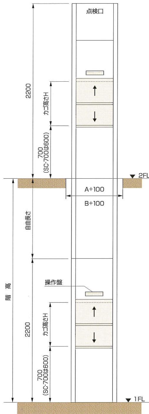
正面図
