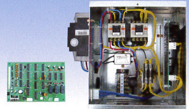
制御盤/基板
