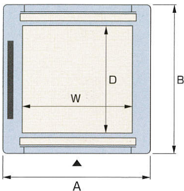
貫通型
